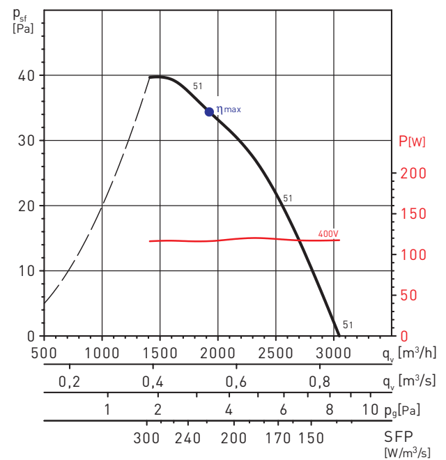
HCBT/6-400/H
