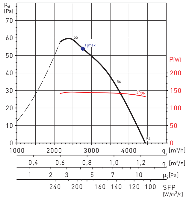
HCFT/6-450/H
