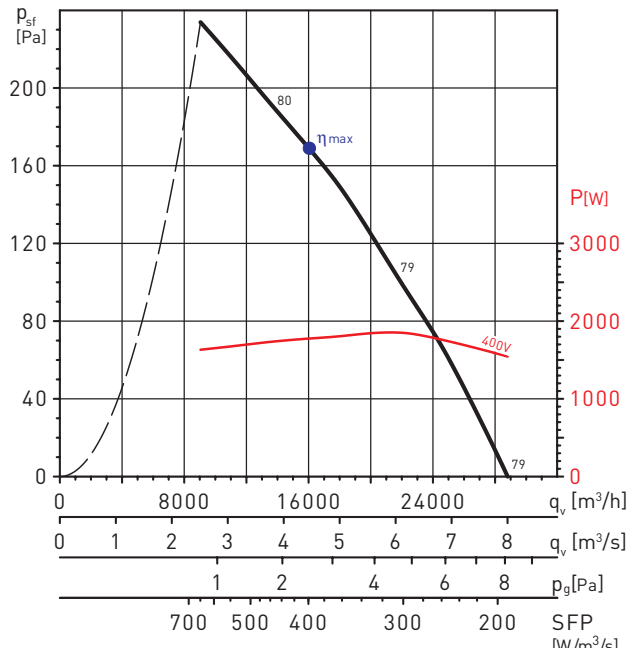
HCBT/6-1000/L
