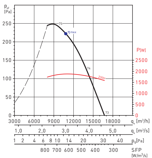
HCBB/4-630/H
