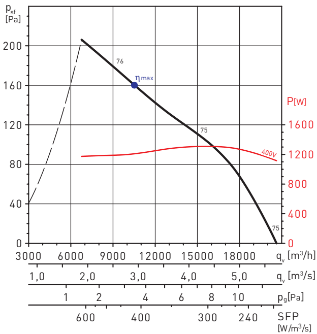
HCBT/6-800/H
